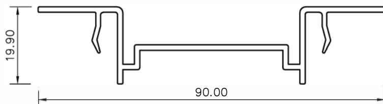
Perfil cerradero marco (hoja corredera)
