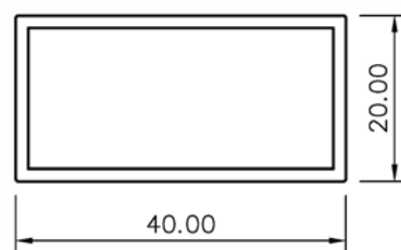
Perfil cabecero
