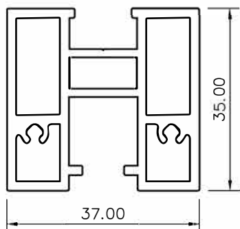
Perfil horizontal hoja
