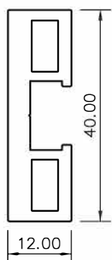
Perfil vertical hoja
