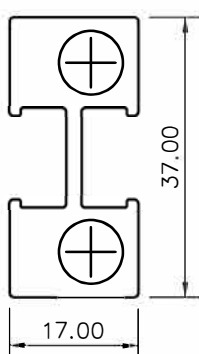
Perfil divisor horizontal
