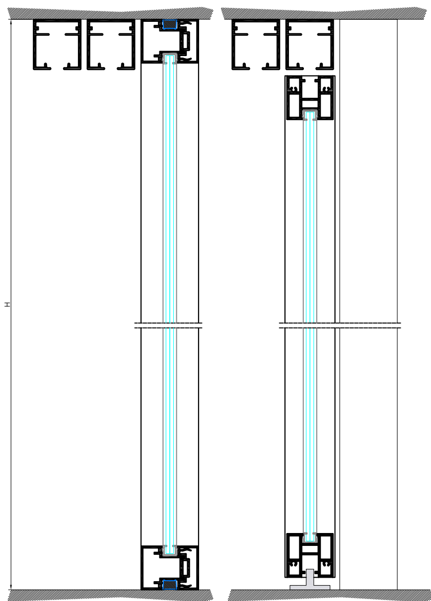
Sección B - B'
