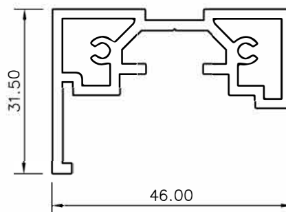
Perfil marco
