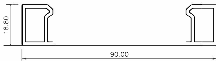
Perfil suplemento cerradero marco (hoja corredera)
