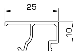
7609 Junquillo 25 mm
