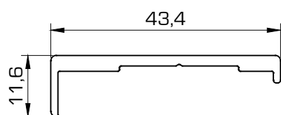
7622 Tapeta hoja centro
