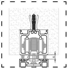
Detalle guía embutida
