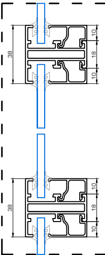
Detalle con junquillo
