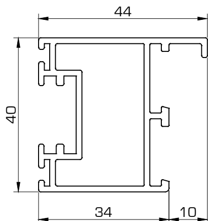
7607 Hoja 40 mm
