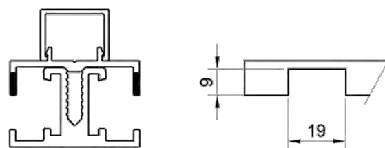
Dimensiones de corte aproximadas (mm)
