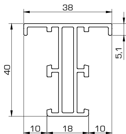
7608 Pilastra junquillo
