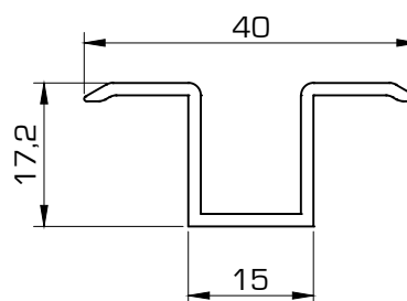
487 Guía inferior encastrada
