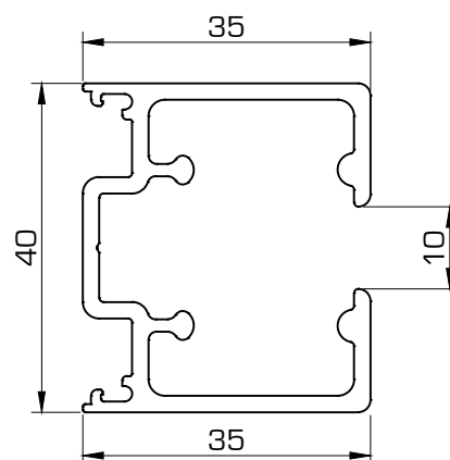
489 Guía superior sin ala
