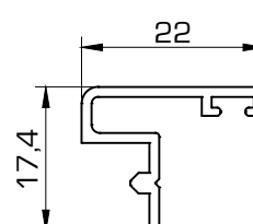
472 Perfil batiente
