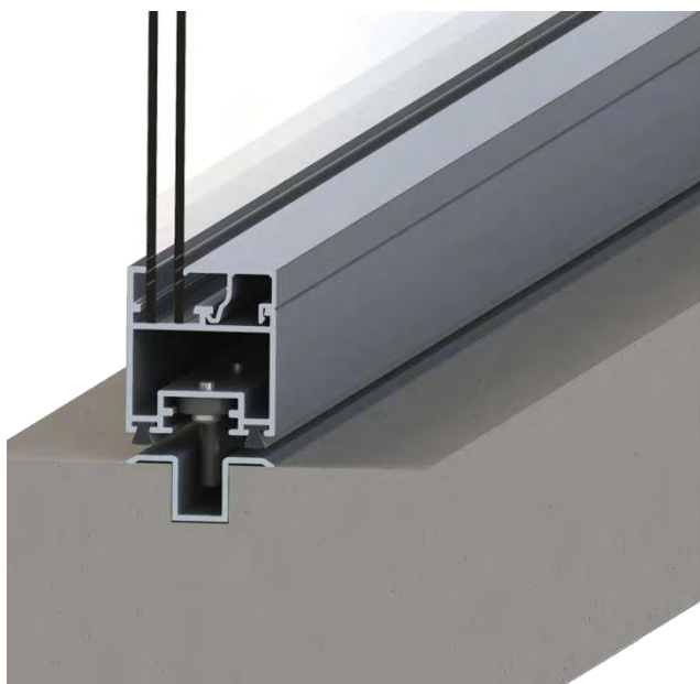
Guía inferior encastrada – Patín guiado
