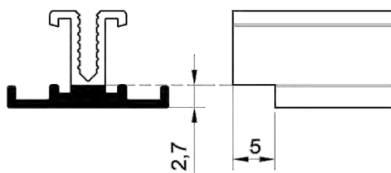
Dimensiones de corte aproximadas (mm)
