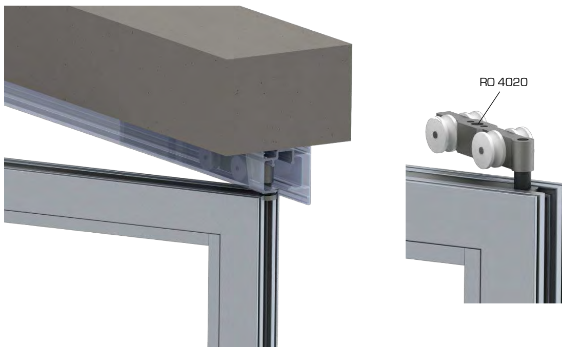
Guía superior con ala – Rodamiento Superior Hojas Pares
