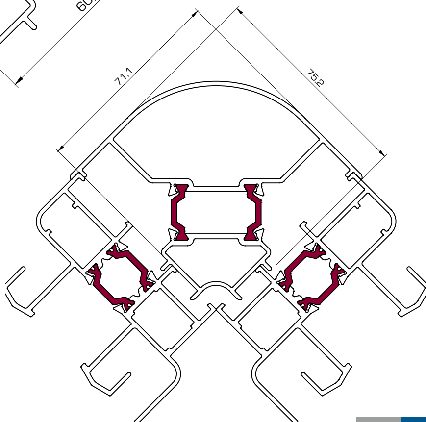
Detalle montaje esquinero 90°
