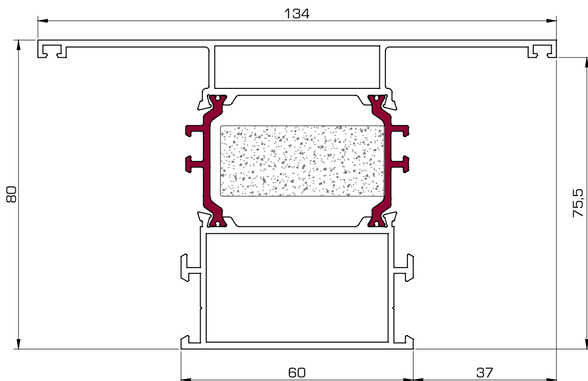
6064 Travesaño 60 mm H.O.
