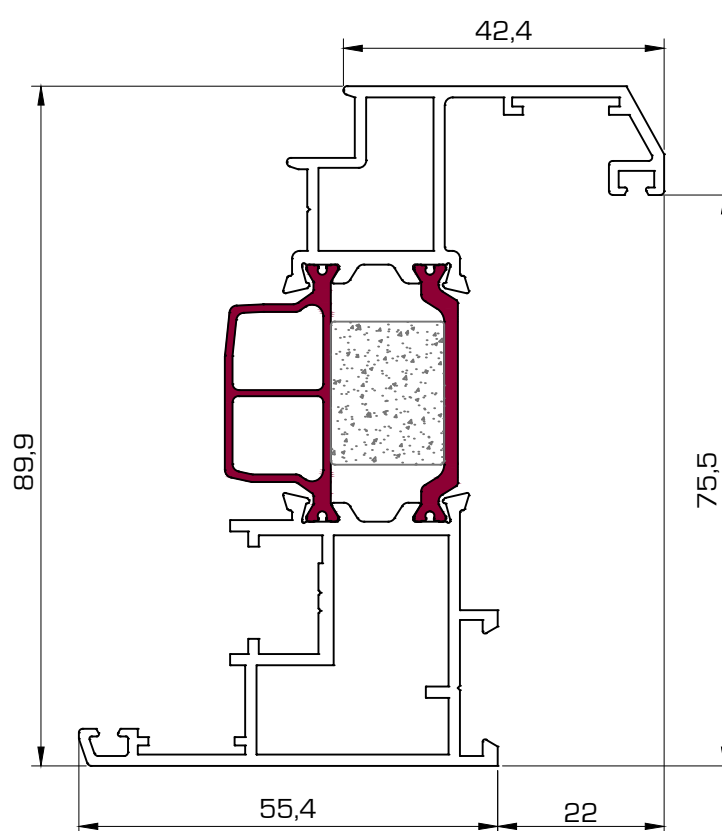
6001 Hoja ventana
