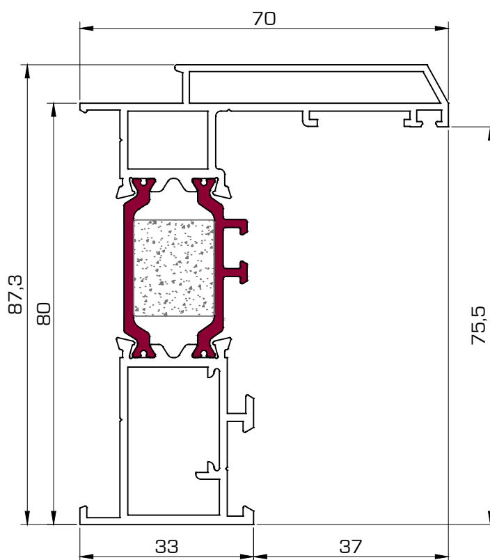
6057 Marco desagüe oculto H.O.
