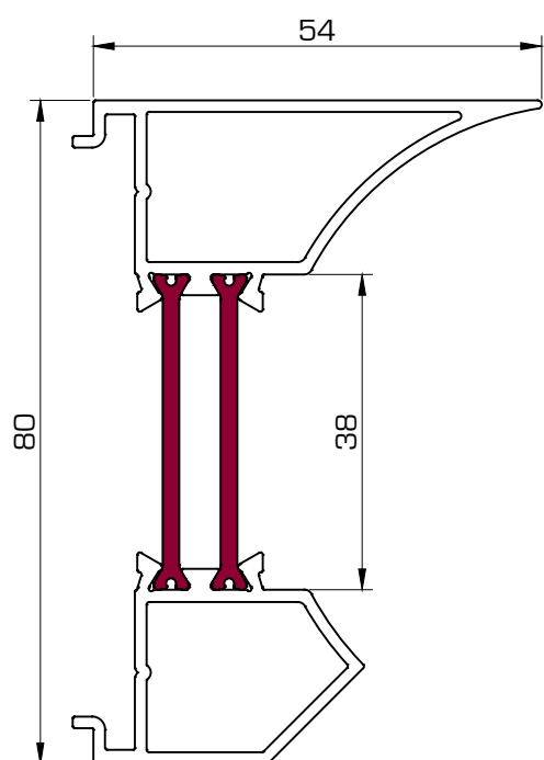
6030 Perfil rótula 80
