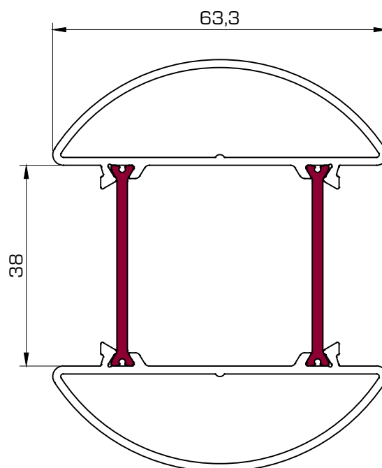
6031 Tubo redondo para perfil rótula 80
