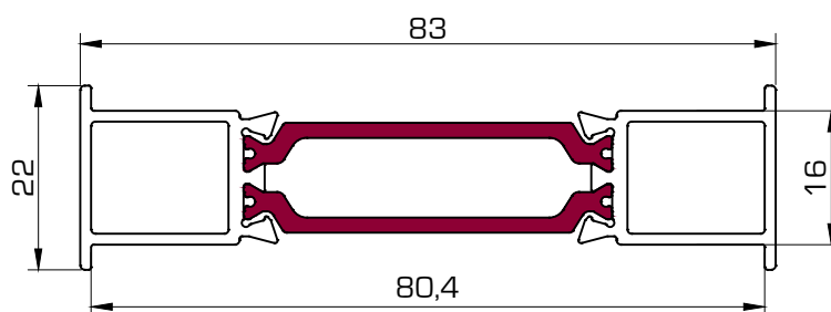
6010 Unión de marcos
