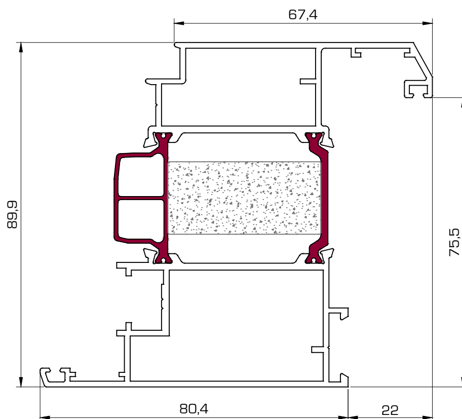
6021 Hoja puerta
