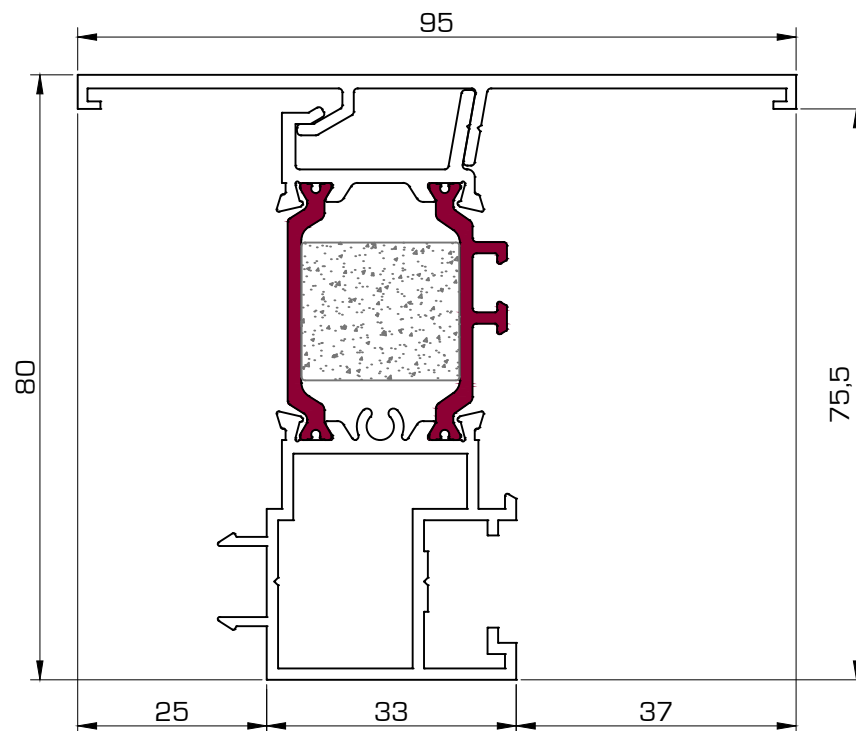
6052 Inversor H.O.
