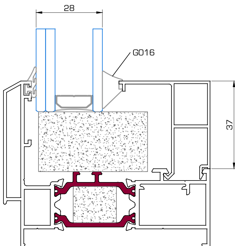
6073 Junquillo 38,5 mm H.O.
