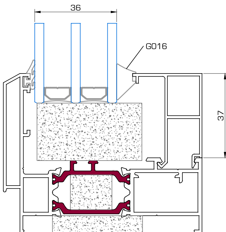
6074 Junquillo 30,5 mm H.O.
