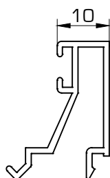
1417 Junquillo 10 mm
