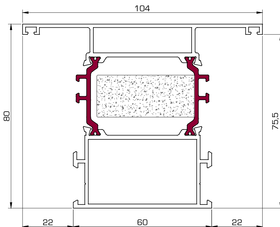
6024 Travesaño 60 mm
