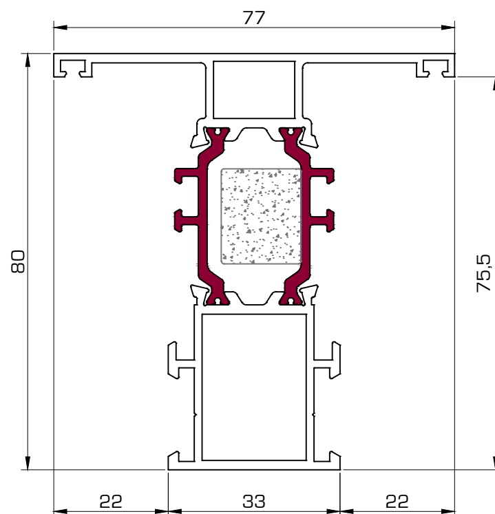
6004 Travesaño 33 mm
