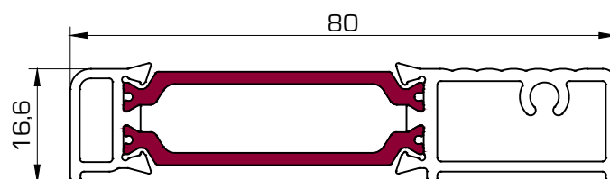
6040 Solera 80 mm
