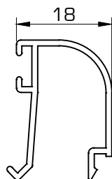
1439 Junquillo 18 mm
