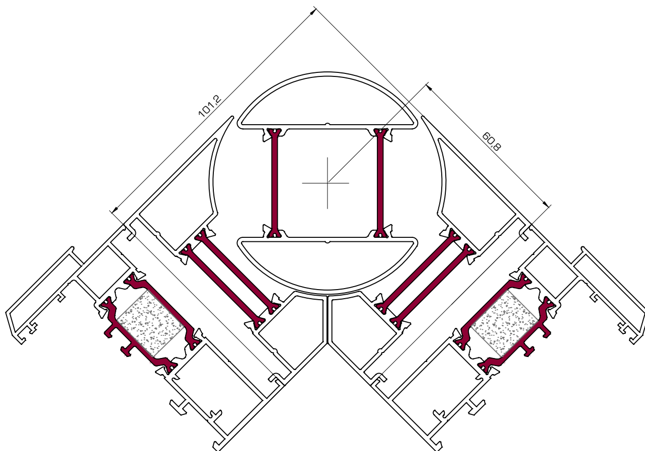
Detalle montaje esquinero rótula
