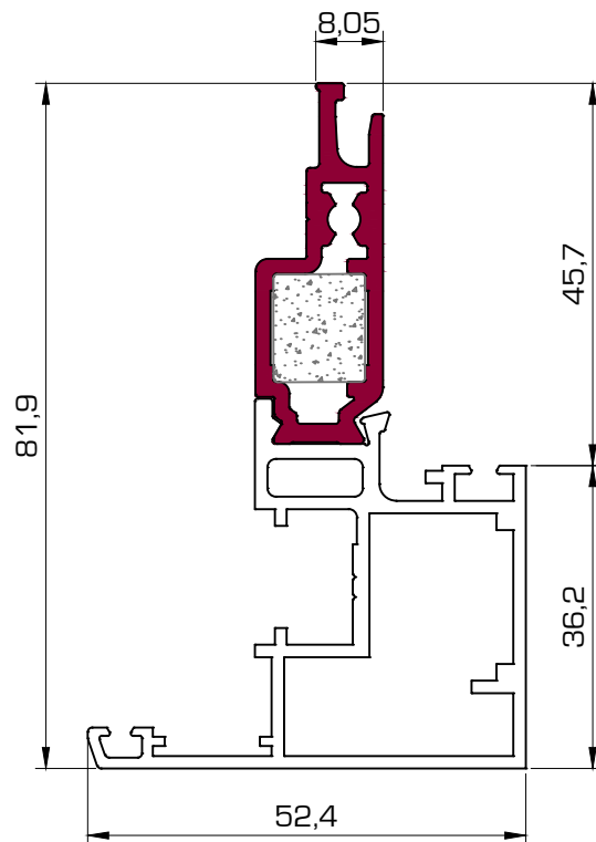
6051 Hoja ventana H.O.
