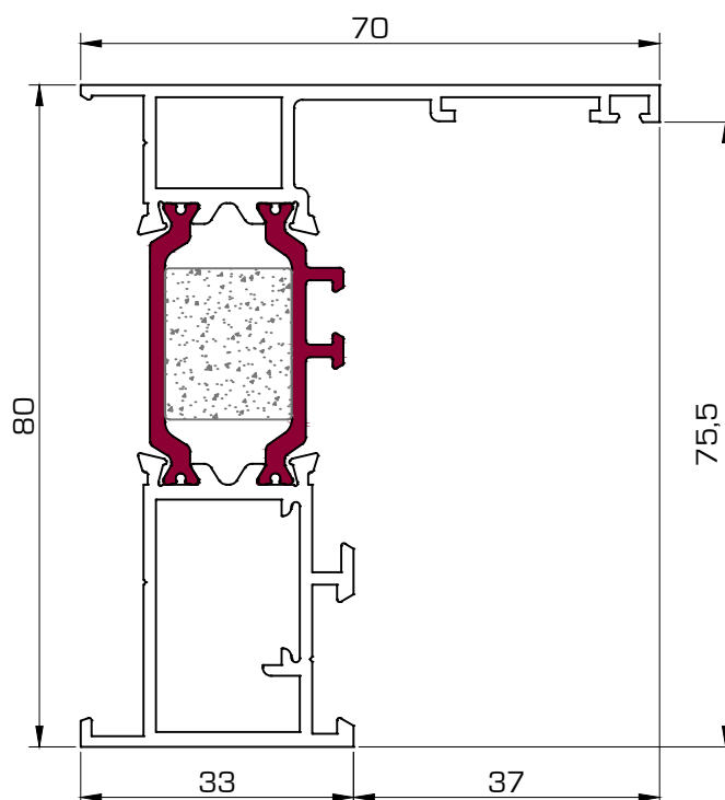
6050 Marco ventana H.O.
