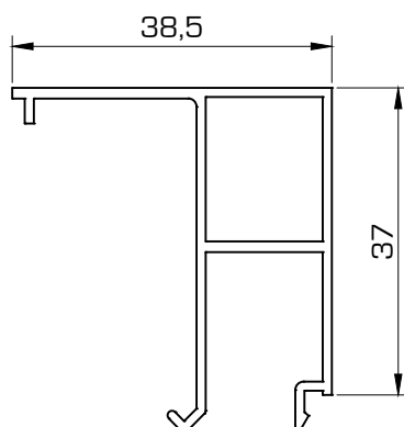
6073 Junquillo 38,5 mm H.O.
