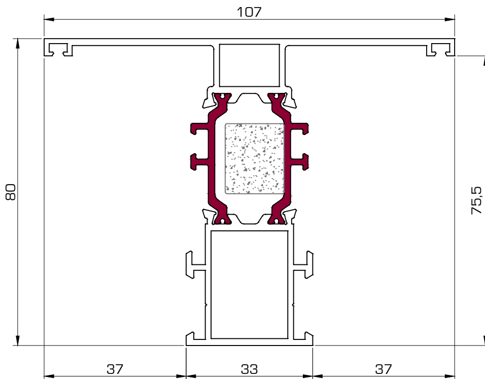
6054 Travesaño 33 mm H.O.
