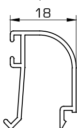
1439 Junquillo 18 mm
