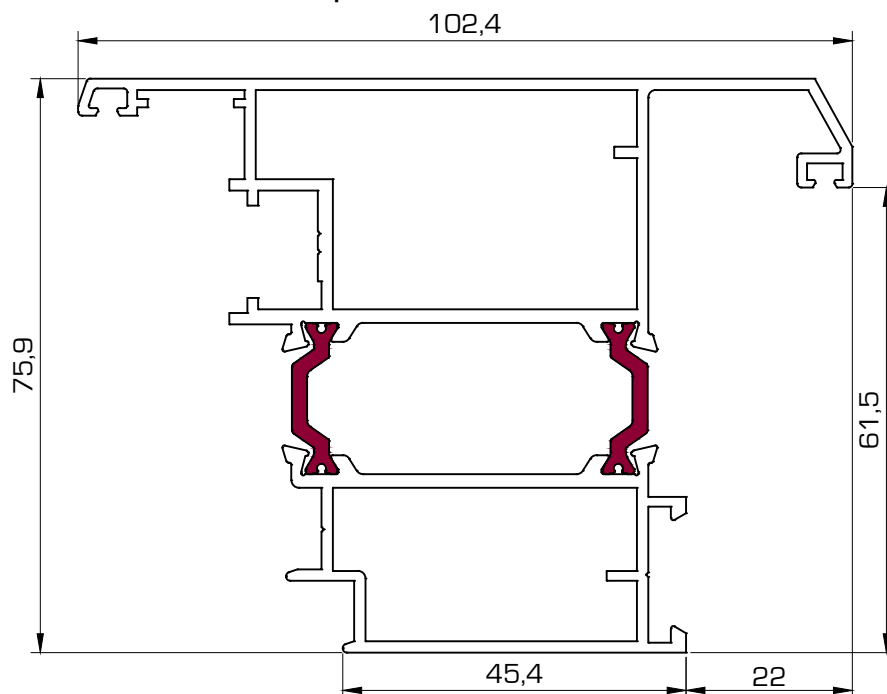
5928 Hoja apertura exterior
