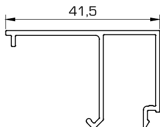
6013 Junquillo 41,5 mm
