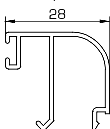
1436 Junquillo 28 mm
