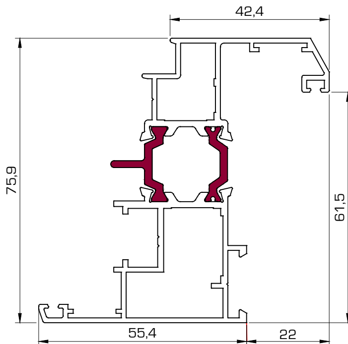
5901 Hoja ventana
