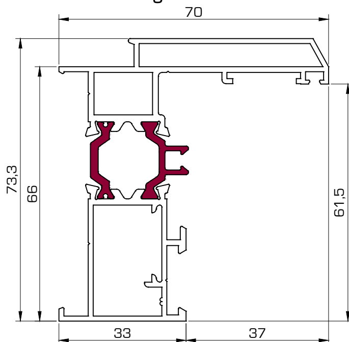
5957 Marco desagüe oculto H.O.
