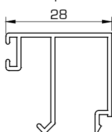
1413 Junquillo 28 mm
