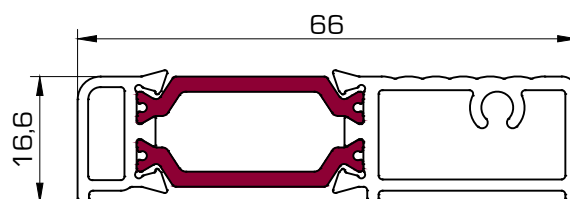
5940 Solera 66 mm
