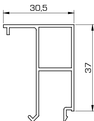
6074 Junquillo 30,5 mm H.O.
