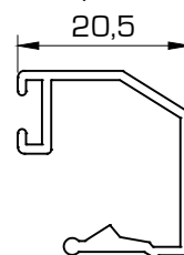
5012 Junquillo 20,5 mm
