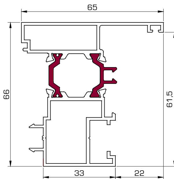
5902 Inversor
