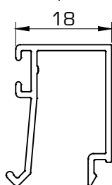
1415 Junquillo 18 mm
