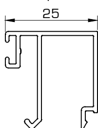
5013 Junquillo 25 mm
