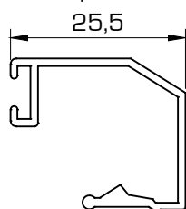
5011 Junquillo 25,5 mm
