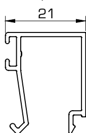
1414 Junquillo 21 mm
