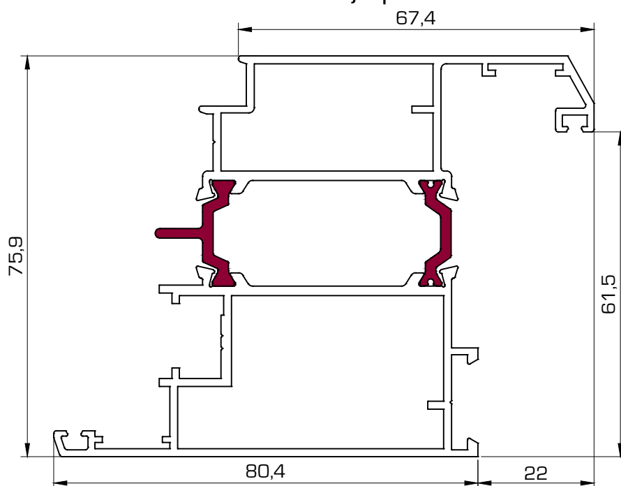
5921 Hoja puerta
