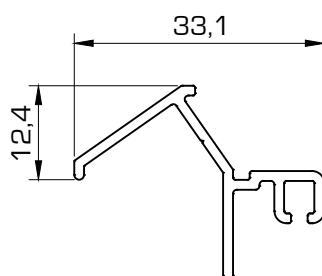
5051 Perfil remate
