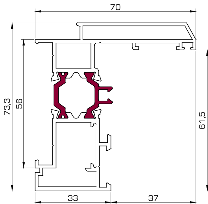
5958 Marco guía desagüe oculto H.O.
