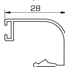
1409 Junquillo 28 mm
