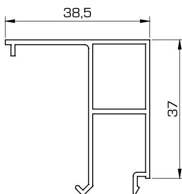
6073 Junquillo 38,5 mm H.O.
