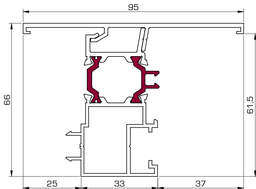
5952 Inversor H.O.
