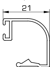
1410 Junquillo 21 mm
