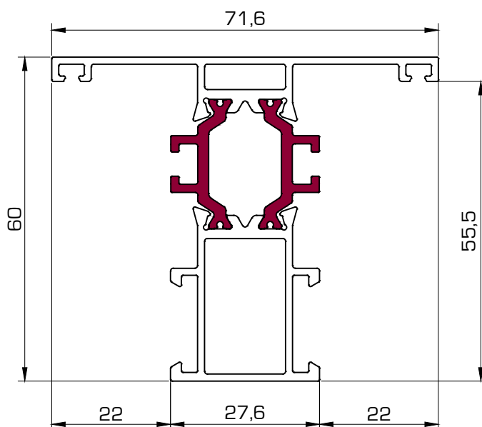
5004 Travesaño pequeño
