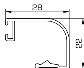
1409 Junquillo 28 mm
