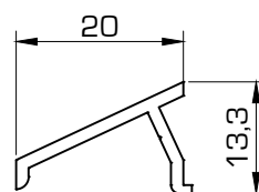
1435 Vierteaguas hoja
