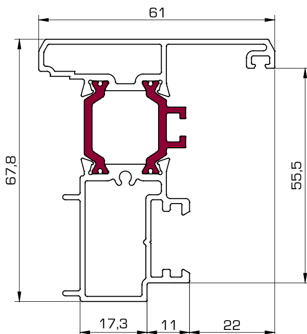
5002 Inversor Euro
