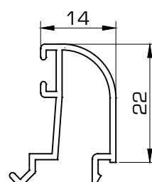
1437 Junquillo 14 mm
