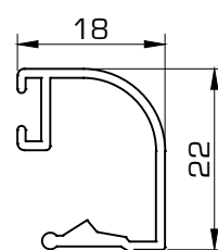
1411 Junquillo 18 mm
