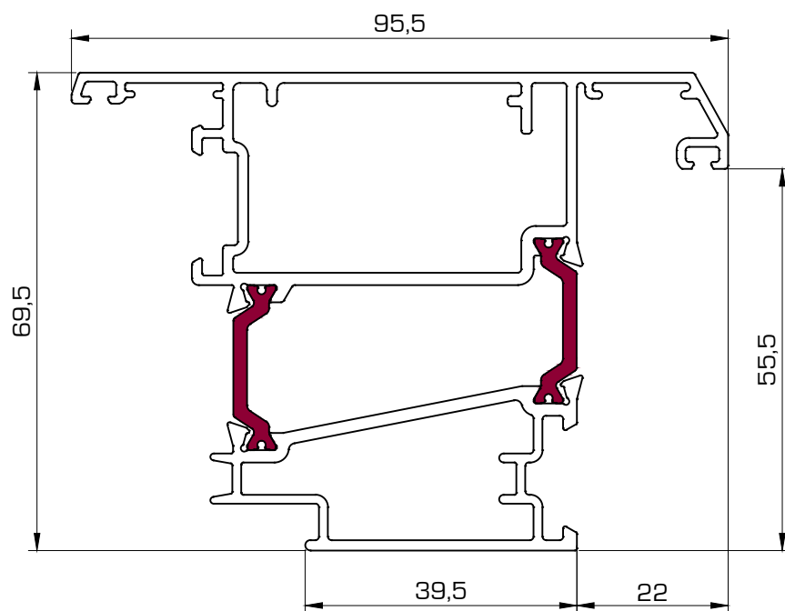
5028 Hoja apertura exterior
