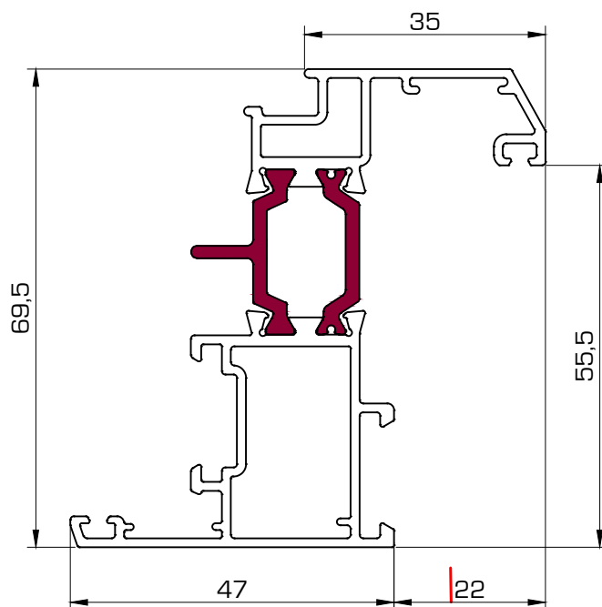
5001 Hoja ventana
