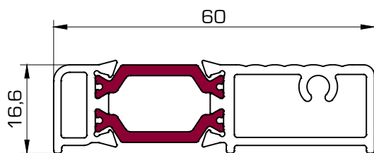
5050 Perfil solera
