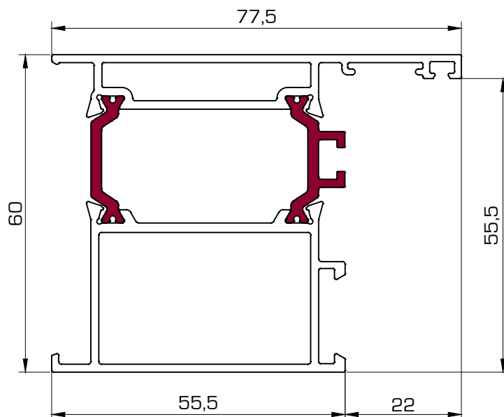
5020 Marco puerta
