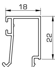
1415 Junquillo 18 mm
