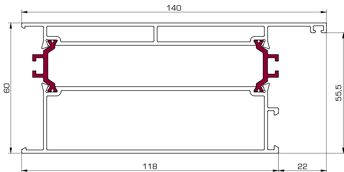
5026 Zócalo
