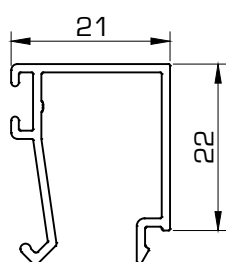
1415 Junquillo 18 mm
