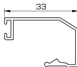
5014 Junquillo 33 mm
