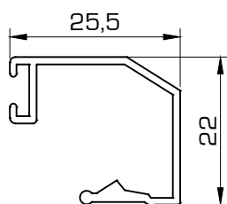
5011 Junquillo 25,5 mm
