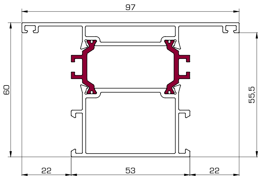
5024 Travesaño grande
