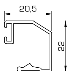
5012 Junquillo 20,5 mm
