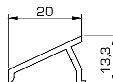
1435 Vierteaguas hoja
