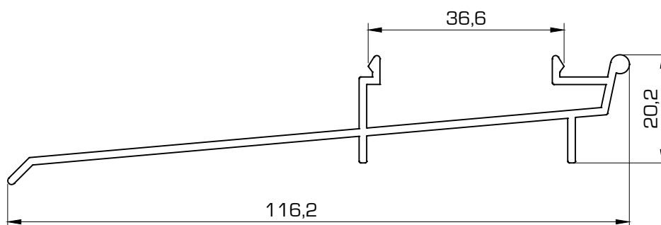
1431 Condensación
