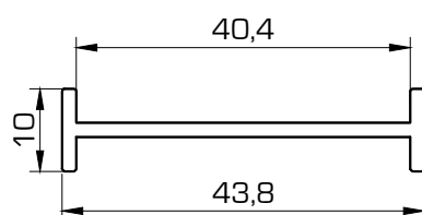
435 Unión Exterior
