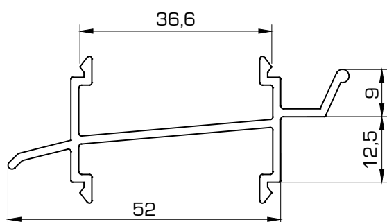
1432 Condensación
