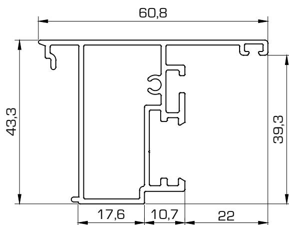
5402 Inversor
