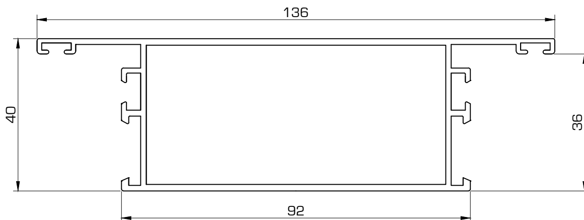
1425 Zócalo central
