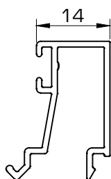
1416 Junquillo 14 mm
