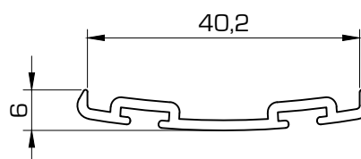
1429 Cortavientos Vaivén
