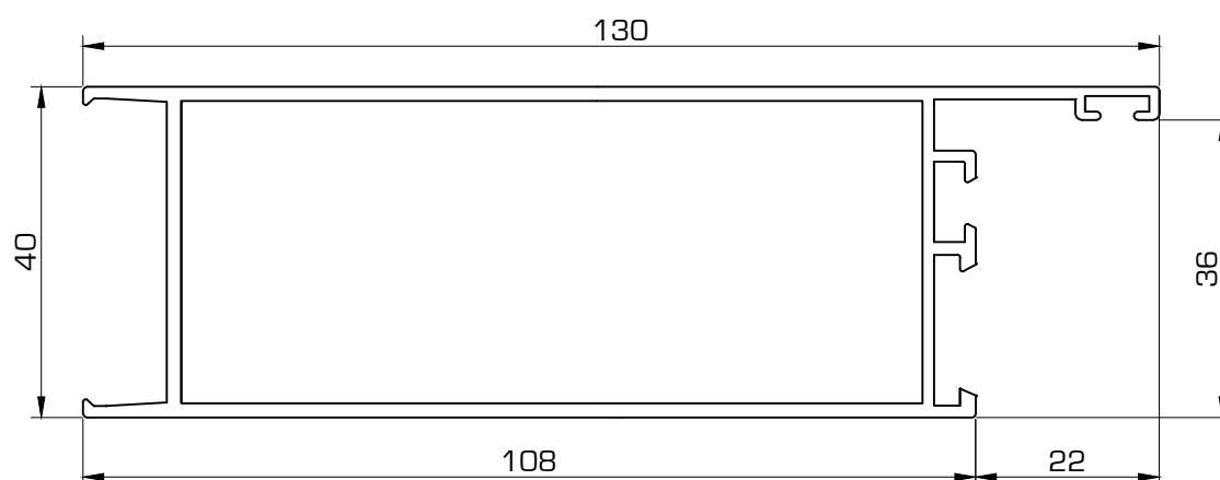
1426 Zócalo inferior
