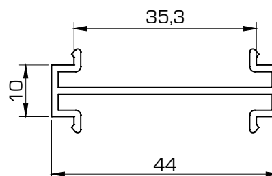
436 Perfil unión
