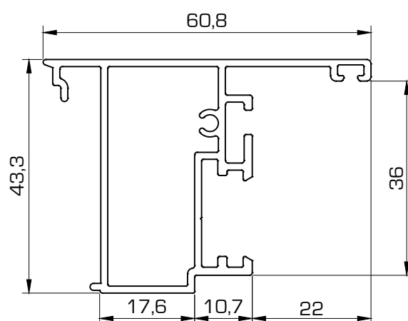
5402 Inversor
