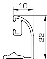
1407 Junquillo 10 mm
