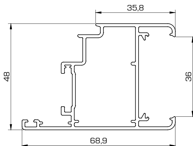
5454 Hoja Mallorca
