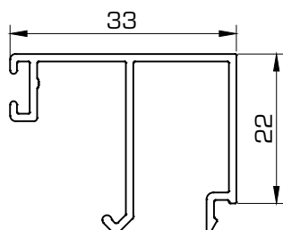
1413 Junquillo 28 mm
