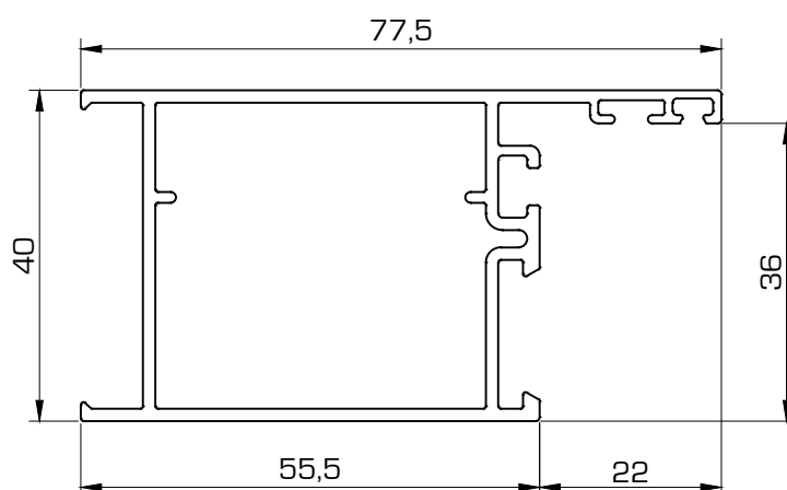
5420 Marco Puerta
