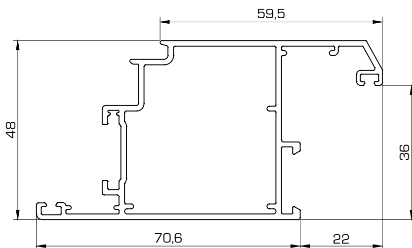
5421 Hoja Puerta
