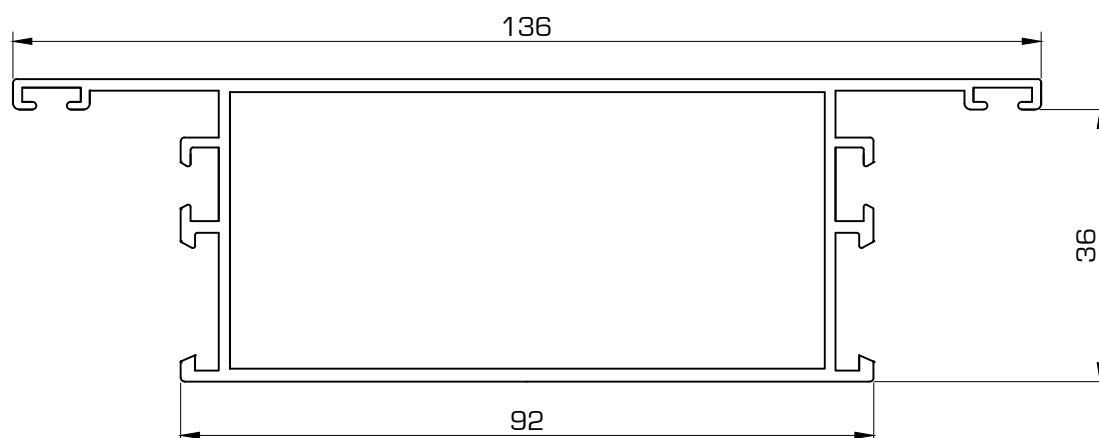
1425 Zócalo central
