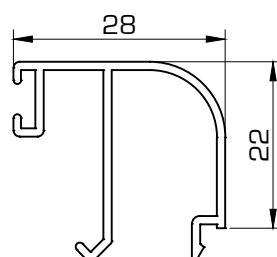
5013 Junquillo 25 mm
