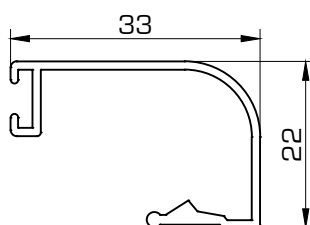
1438 Junquillo 33 mm
