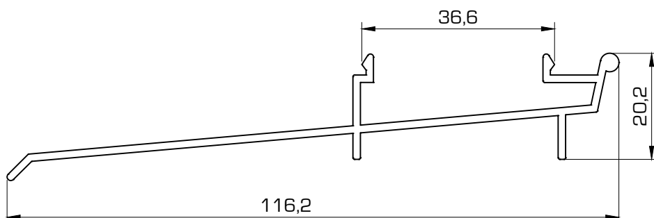
1431 Condensación
