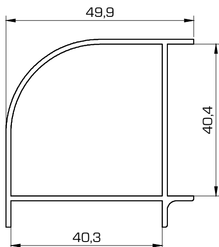
430 Esquinero curvo 90°
