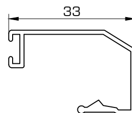
5014 Junquillo 33 mm
