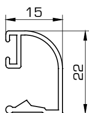
1412 Junquillo 15 mm
