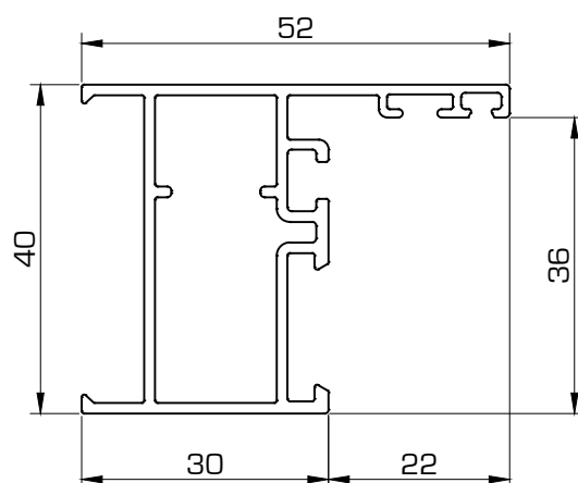
5400 Marco Ventana
