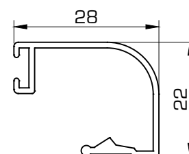
1409 Junquillo 28 mm
