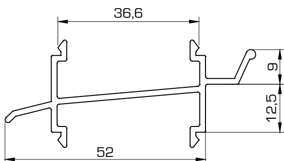
1432 Condensación
