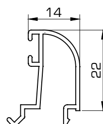
1437 Junquillo 14 mm
