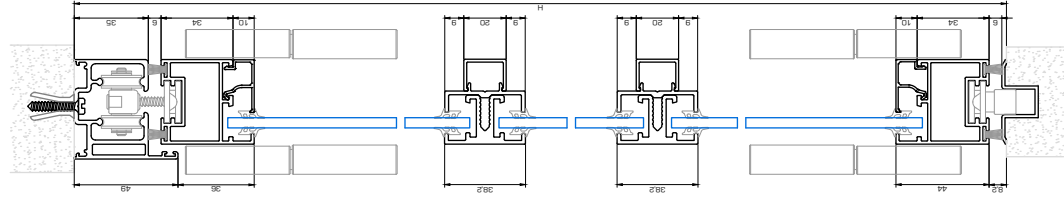
Detalle guía embudida
