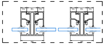
Detalle con jurquillo
