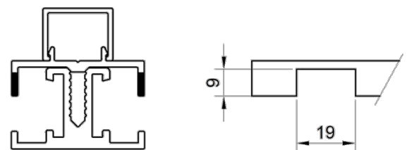
Dimensiones de corte aproximadas (mm)
