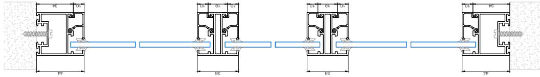
Detalle con junquillo
