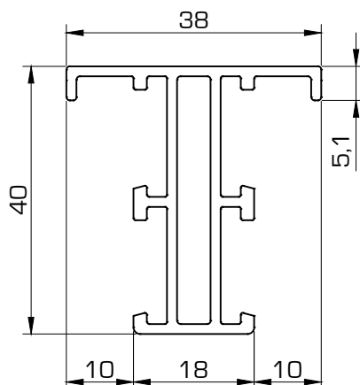
7608 Pilastra junquillo
