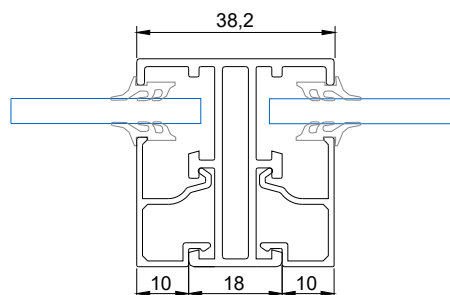
Solución ajunquillada
