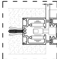
Detalle guía embutida
