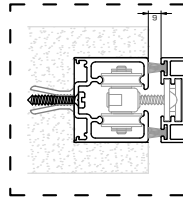
Detalle guía embudida
