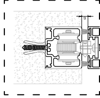
Detalle guía embutida
