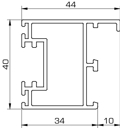
7607 Hoja 40 mm
