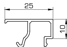
7609 Junquillo 25 mm
