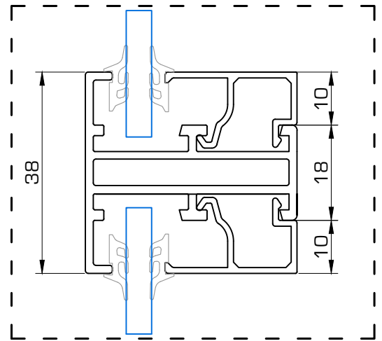
Detalle con junquillo
