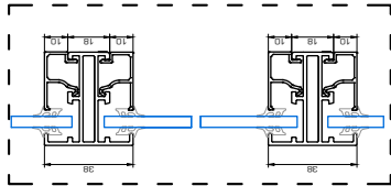
Detalle con junquillo
