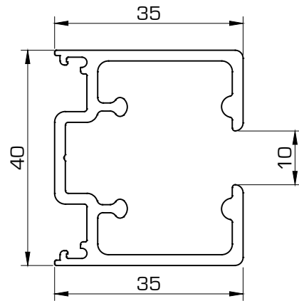
489 Guía superior sin ala
