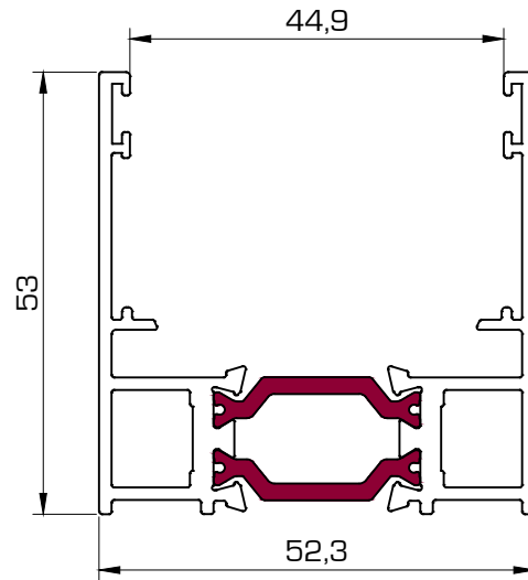
1008 Marco monocarril minimalista
