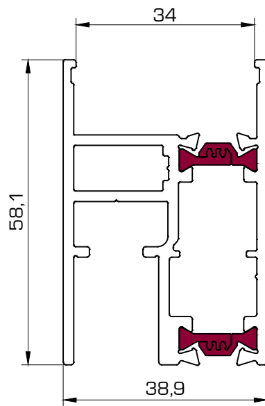
1021 Hoja lateral para cerradura (BIMETAL)
