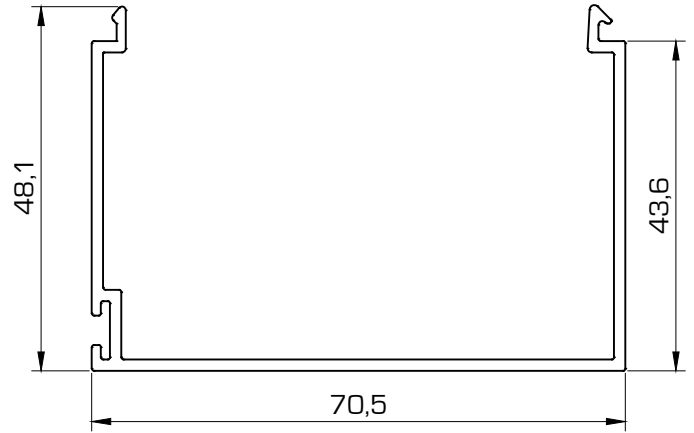
1018 Tapeta galandage
