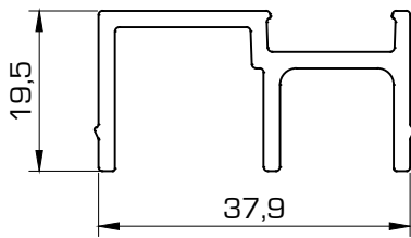
1010 Suplemento carril rodadura
