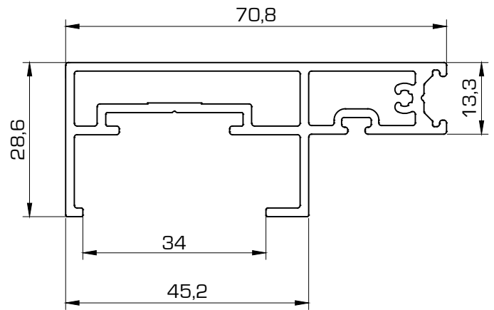
1013 Pilastra fijo integrado
