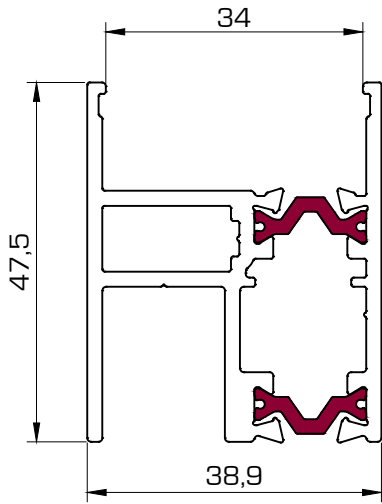
1007 Hoja lateral / inferior
