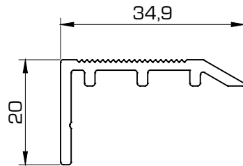
1022 Solape deslizante solera
