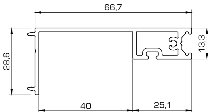
1002 Hoja centro
