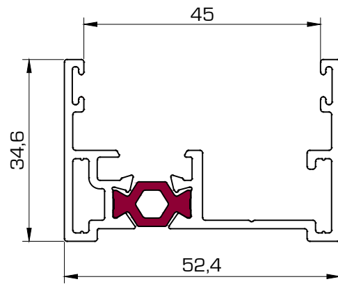
1009 Perfil unión 4 hojas
