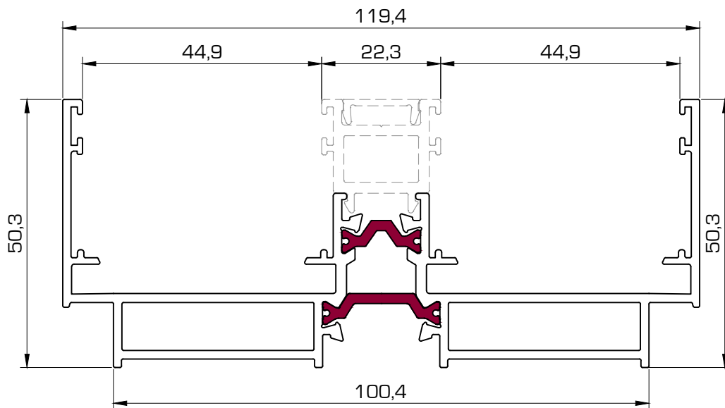
1000 Marco 2 carriles minimalista
