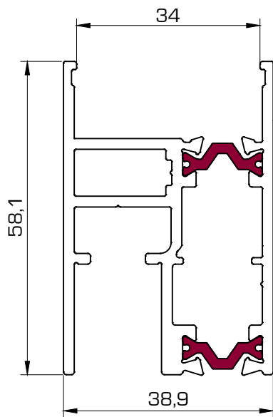
1027 Hoja lateral para cerradura
