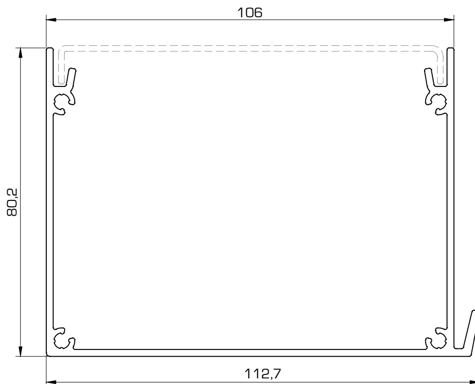
1019 Canal portarejilla
