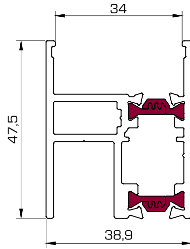
1001 Hoja lateral / inferior (BIMETAL)
