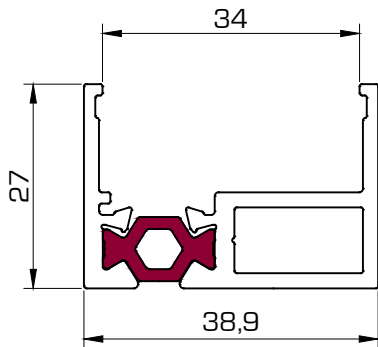
1005 Hoja centro / superior
