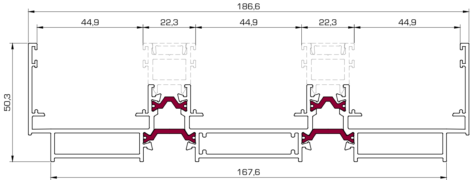
1006 Marco 3 carriles minimalista
