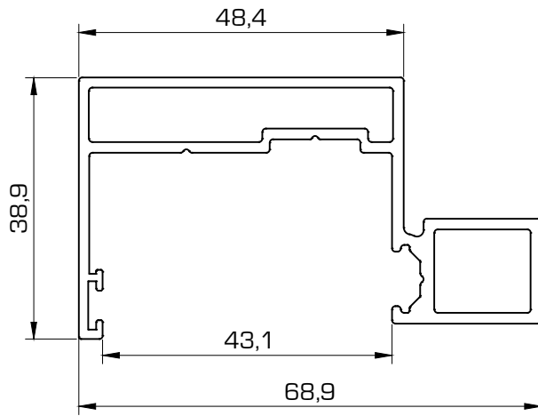
1014 Unión Marco en esquina
