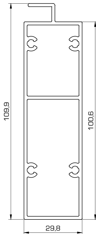
1020 Suplemento carril embutido
