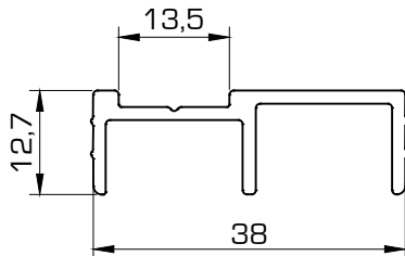
1012 Suplemento lateral cerradero
