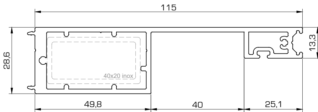
1003 Hoja centro refuerzo
